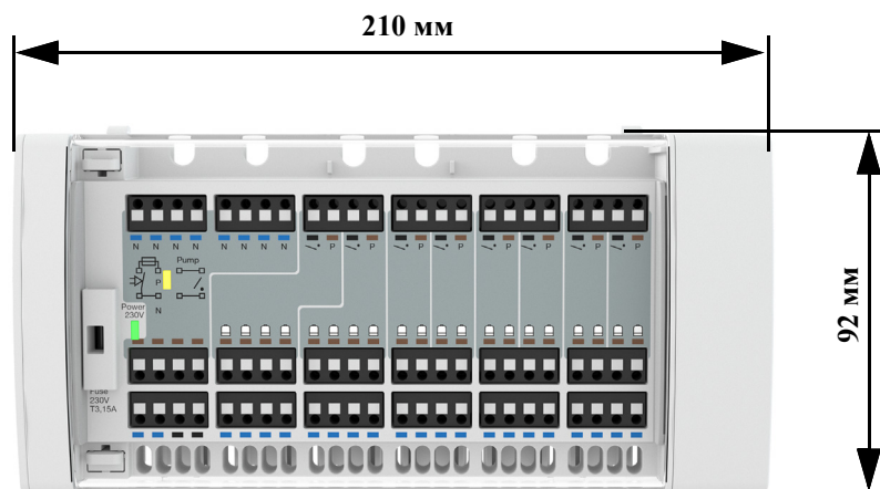
Рисунок 1: Размеры изделия
